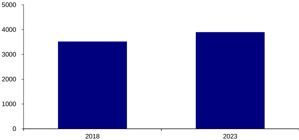
图：白云鄂博矿稀土储量（亿吨，REO）
